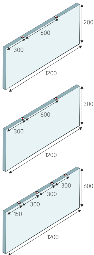
Вертикальное крепление
