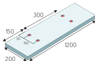
Горизонтальное крепление
